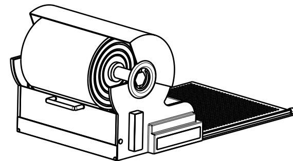
Vue isométrique Echelle : 1:10
